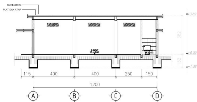
POTONGAN B SKALA 1 : 100 04 AR-04
