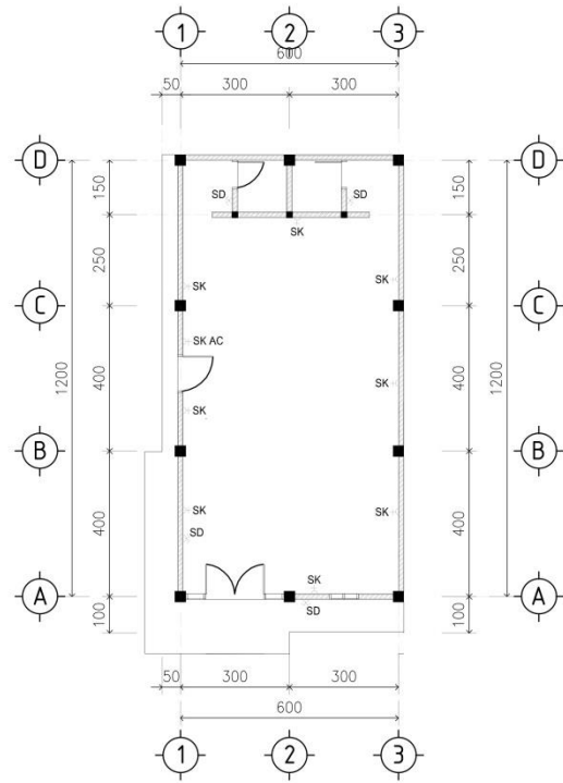
DENAH STOP KONTAK 20 SKALA 1 : 100 ME 20
