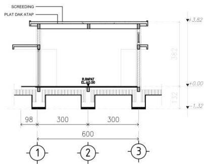
POTONGAN A SKALA 1 : 100 04 AR-04
