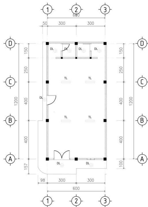
DENAH TITIK LAMPU 19 SKALA 1 : 100
